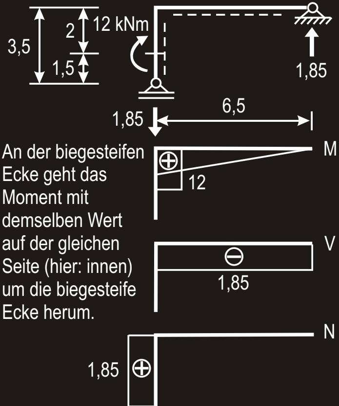
GEKNICKTE TRÄGER
